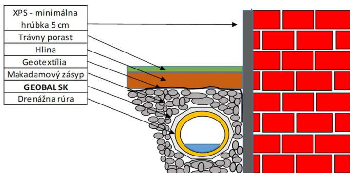
Izolácia základov
