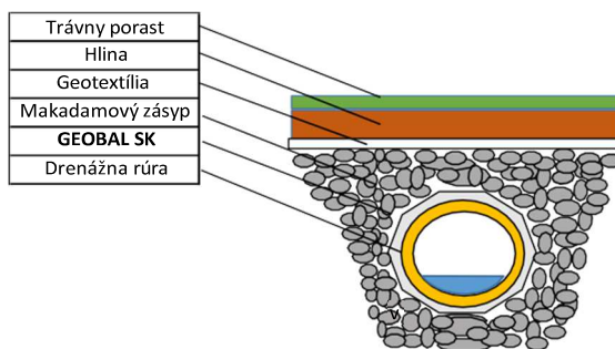
Lineárne odvodnenie
